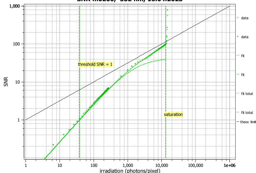
SNR m0200, 532 nm, 16.04.2023
